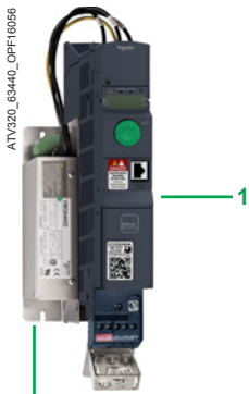
VW3A4422 + ATV320U04N4B
