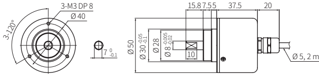
Axial cable type (IP64)
